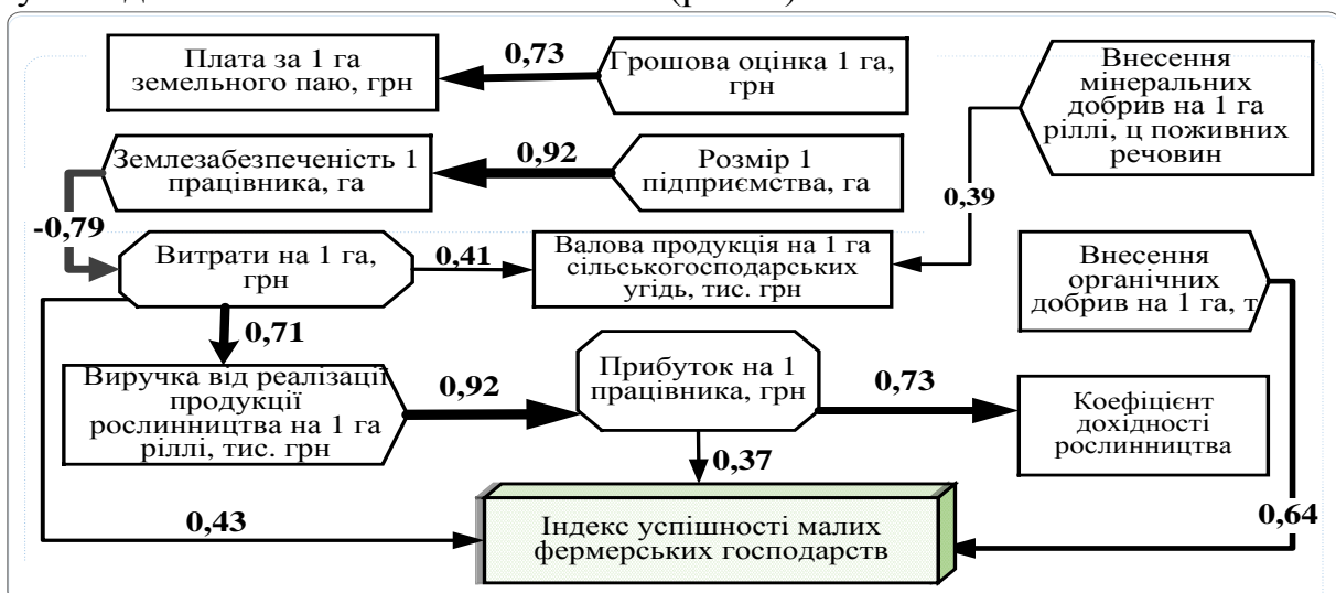
Рис. 3. Шляхова діаграма стандартизованої багатофакторної регресії між показниками успішності малих фермерських господарств
